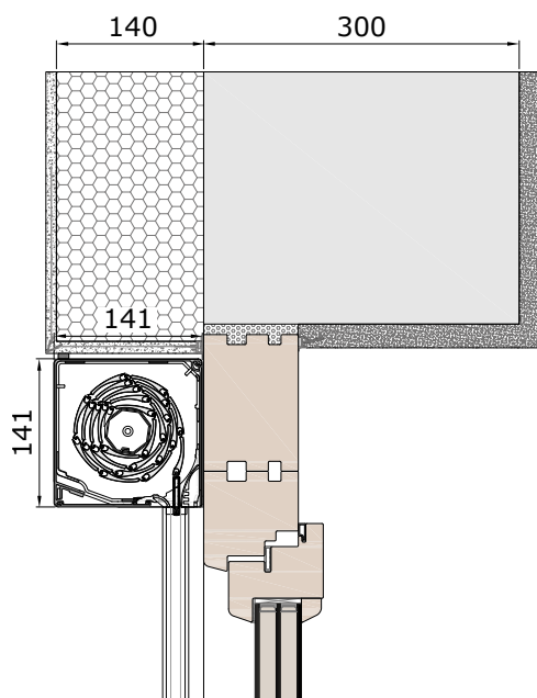
Hőszigeteléssel és tokmagasítással. VORO SE.
