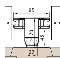
ED85V vezetősín
