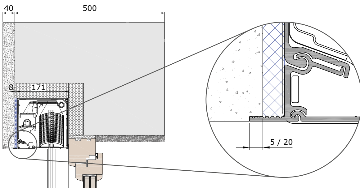
Bevakolásra alkalmas kivitel. Vakolósín szélessége: 5 és 20 mm (alapkivitel: 5 mm)
