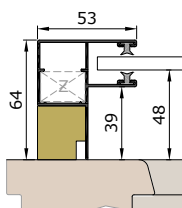
Termikusan leválasztott KD53VT vezetősín
