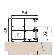
KR54V vezetősín
