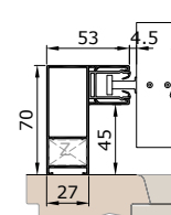
ED53V vezetősín
